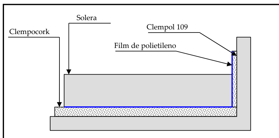
Detalle instalación del CLEMPOCORK
